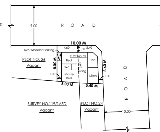
SITE PLAN SCALE - 1:250
