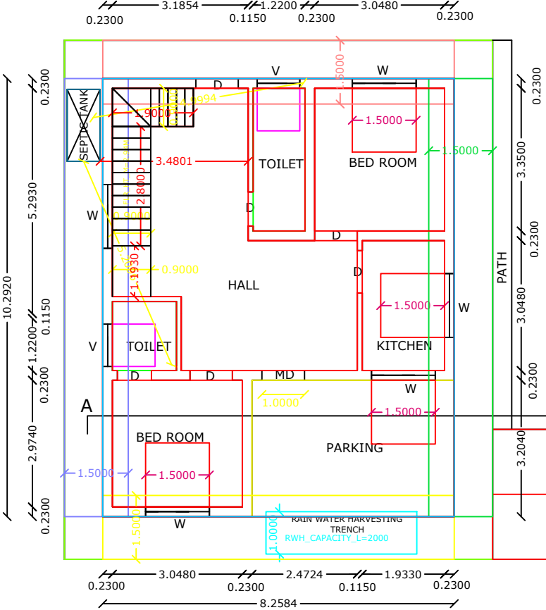
PRO G.FLOOR PLAN
