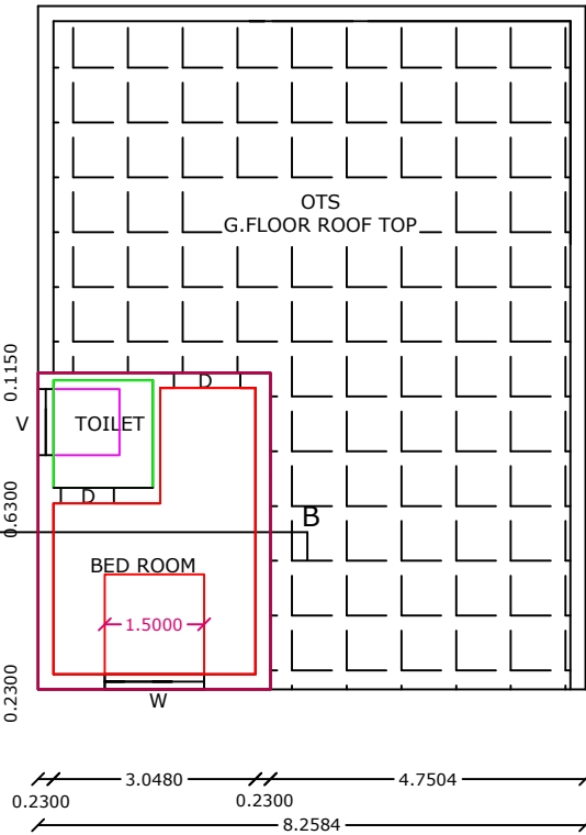
PRO F.FLOOR PLAN
