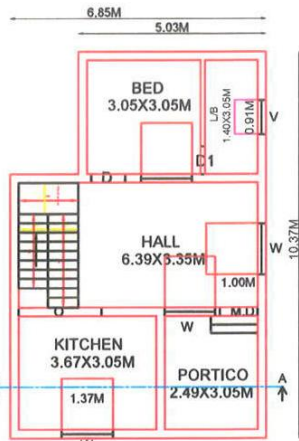
PRO. G.F. PLAN
