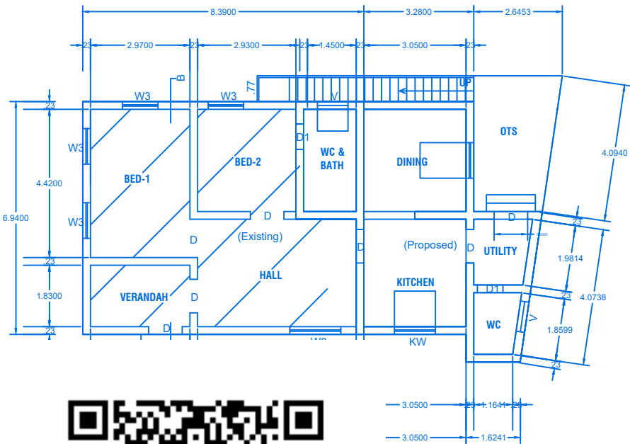
DR PLAN
