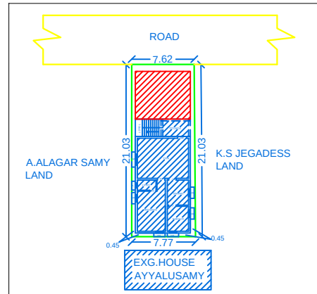
SITE PLAN (Scale 1:400)
