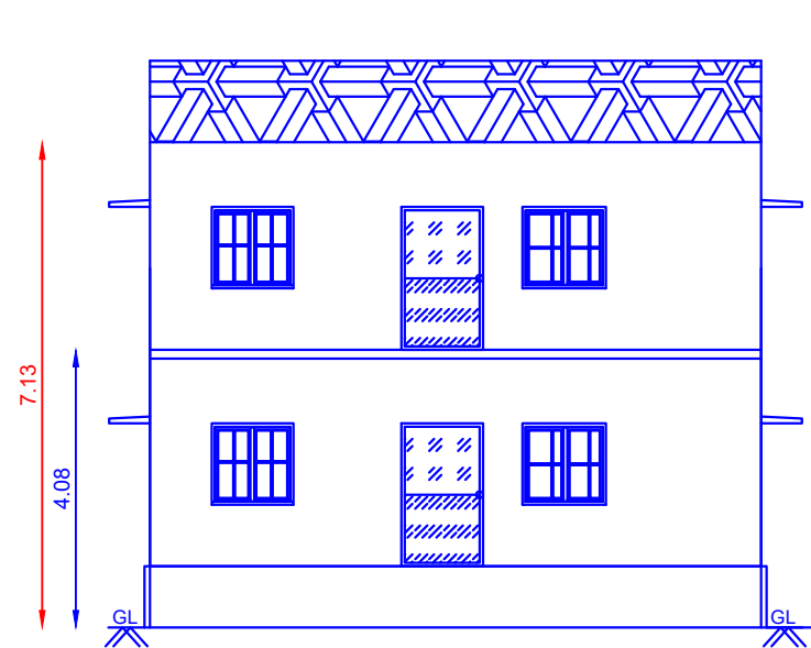
ELEVATION
