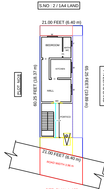
SITE PLAN 1:100
