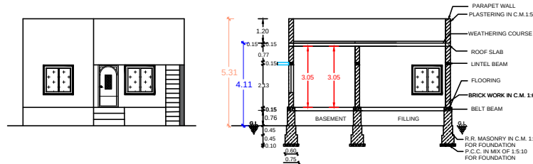
ELEVATION
