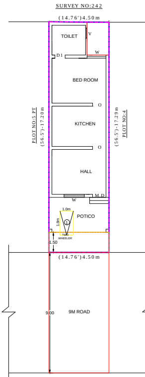
SITE PLAN (SCALE : - 1:100)
