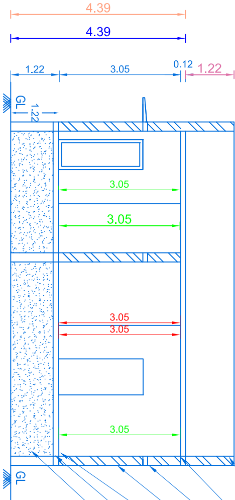
SECTION A-A
