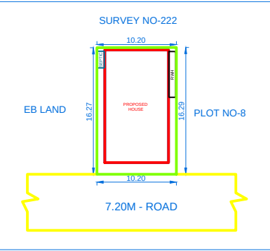
SITE PLAN (Scale 1:400)
