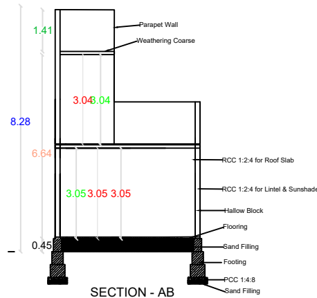
SECTION - AB
