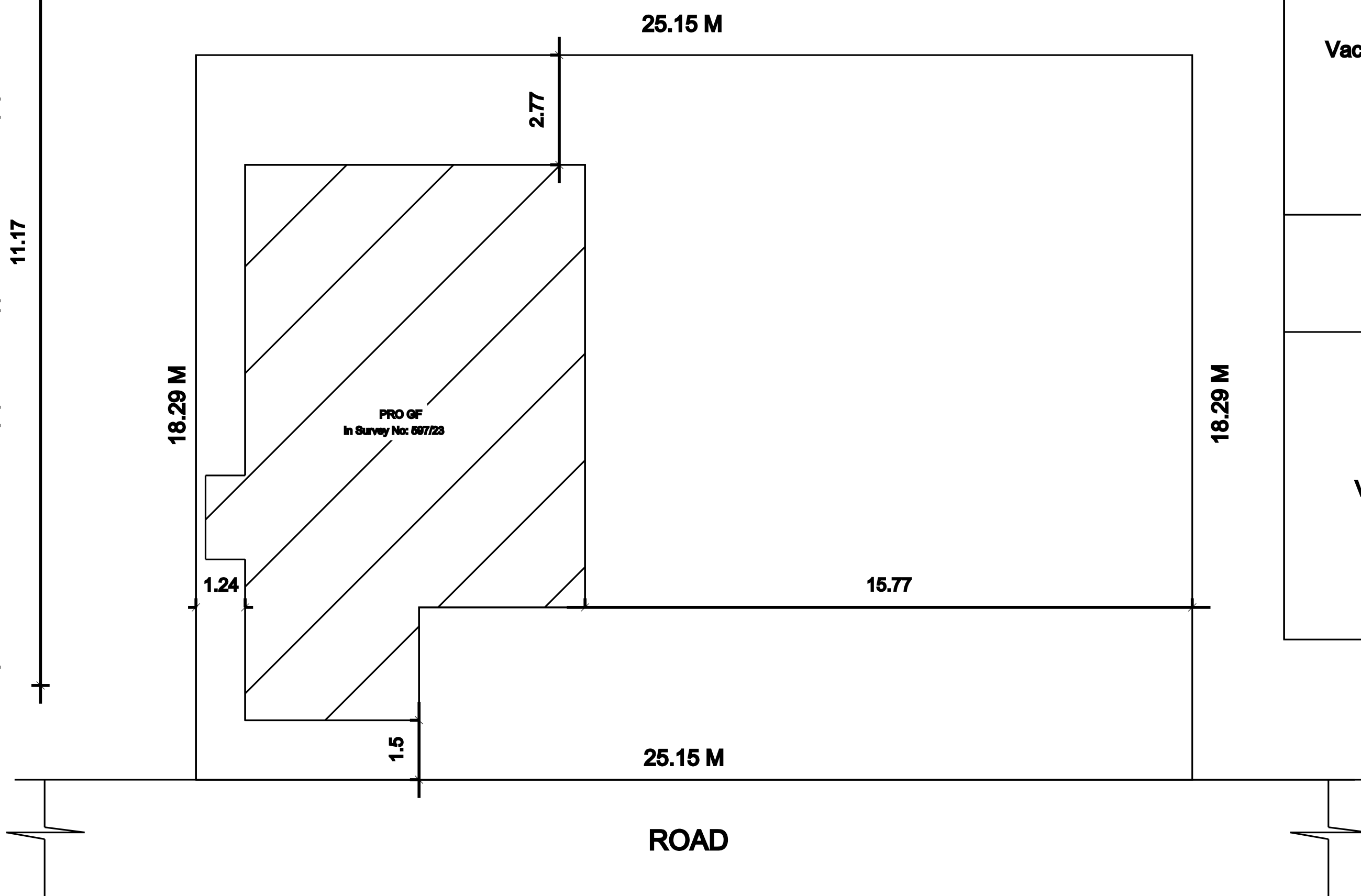
SITE PLAN (1:200)
