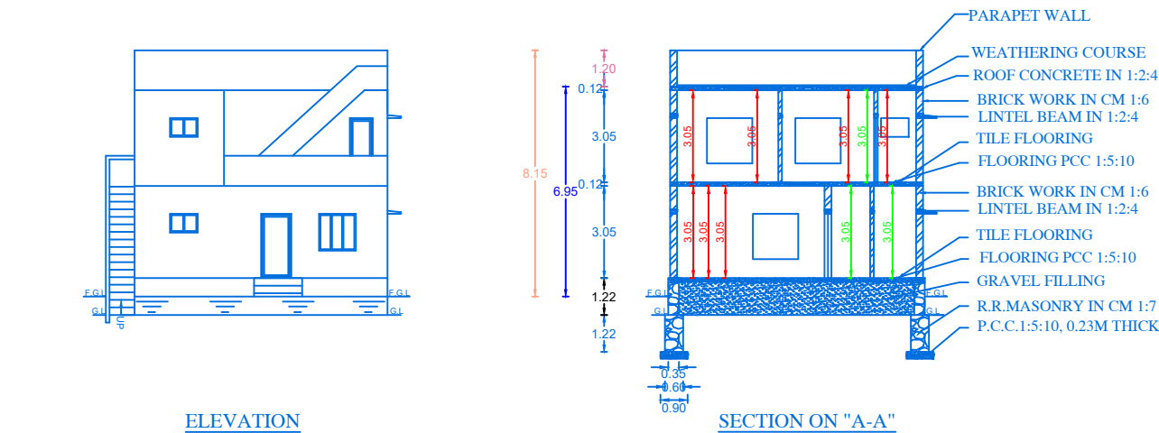
ELEVATION
