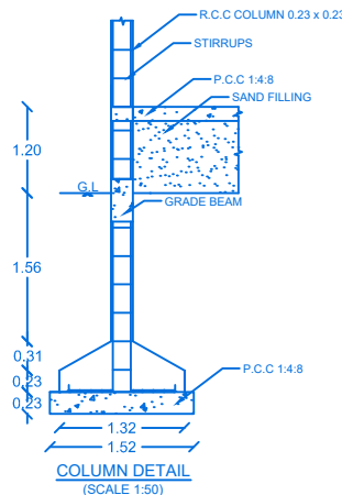
COLUMN DETAIL (SCALE: 1:50)
