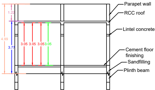
SECTION - AB
