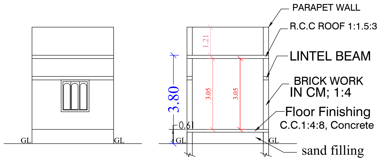
ELEVATION
