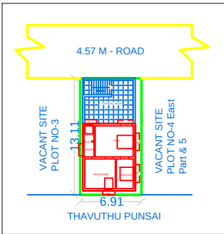
SITE PLAN (Scale 1:400)
