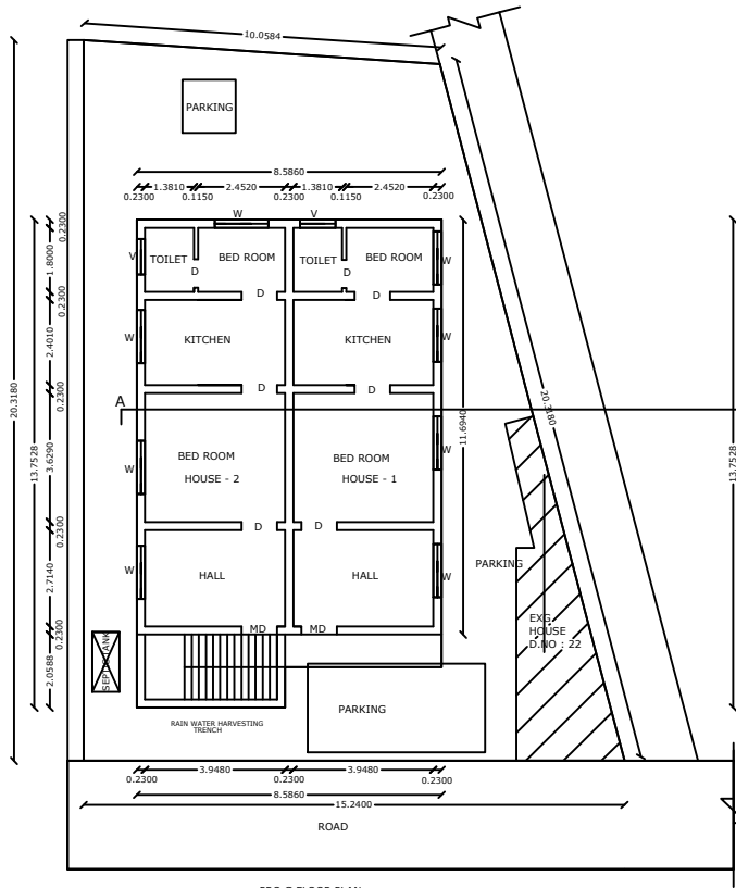
PRO G.FLOOR PLAN
