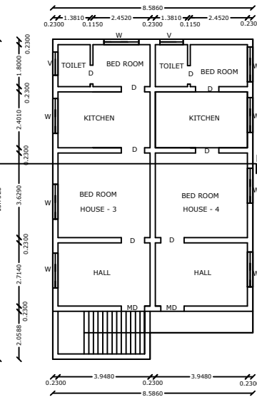
PRO F.FLOOR PLAN
