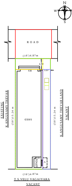
SITE PLAN SCALE : - 1:100
