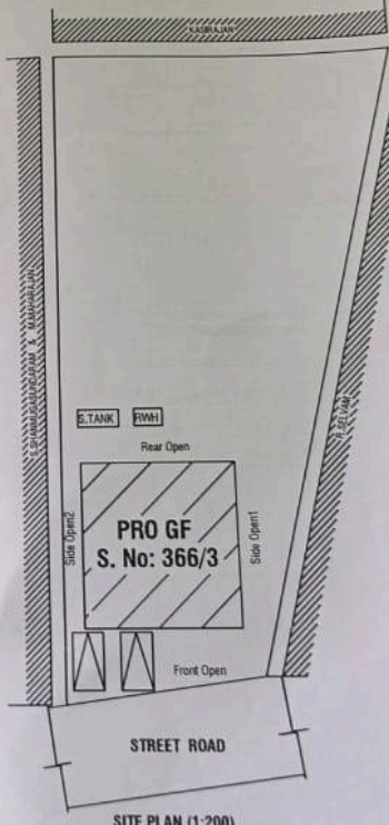
SITE PLAN (1:200)
