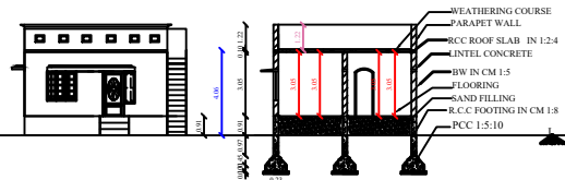
ELEVATION
