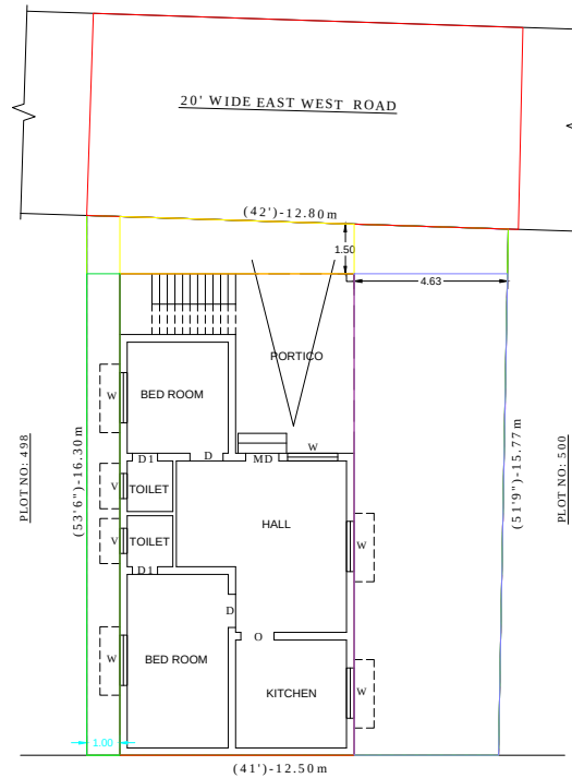
SURVEY NO: 190 SITE PLAN (SCALE : - 1:100)
