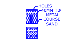
R.W.H. CAPACITY, L = 2000LTRS
