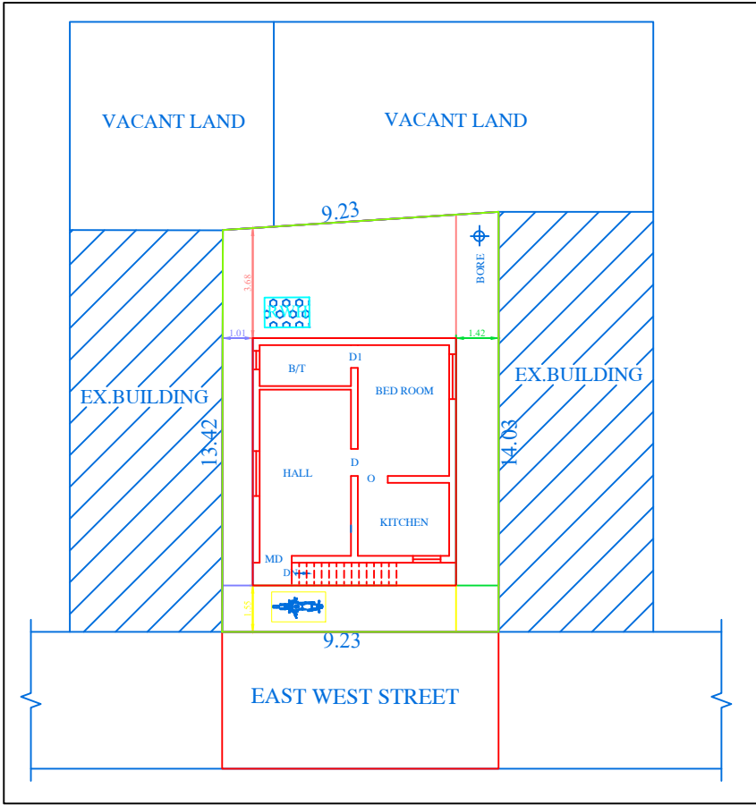
SITE PLAN(Scale 1 : 100)
