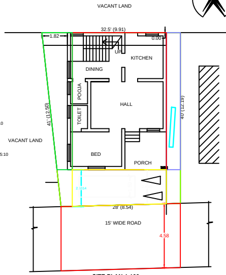
SITE PLAN 1:100
