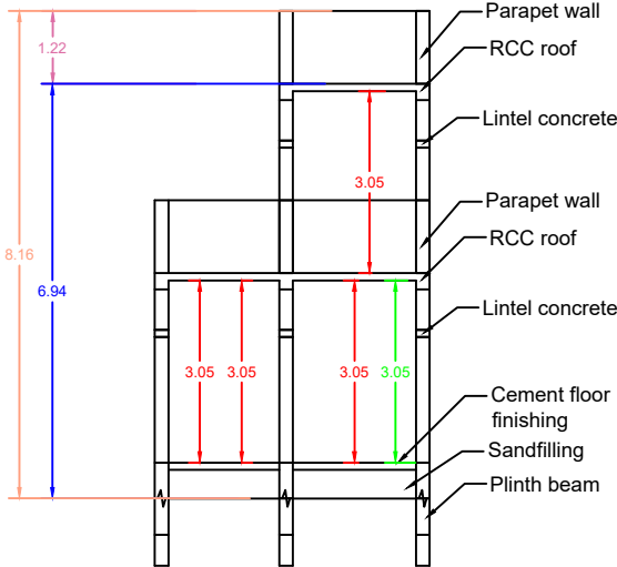
SECTION - AB
