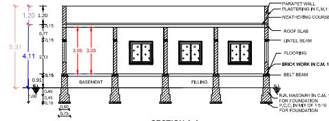
SECTION A-A
