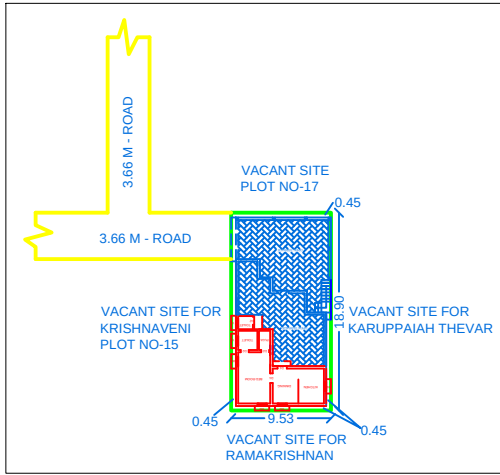
SITE PLAN (Scale 1:400)
