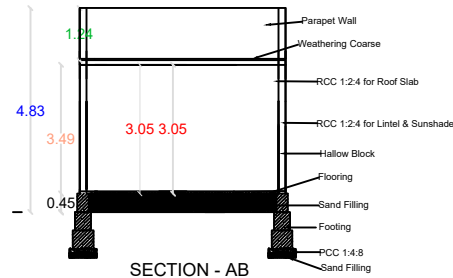
SECTION - AB
