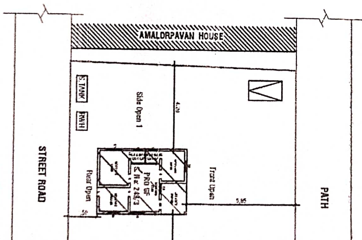
SITE PLAN (1:200)
