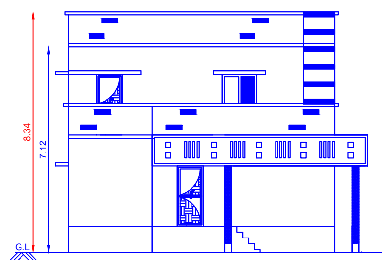
ELEVATION
