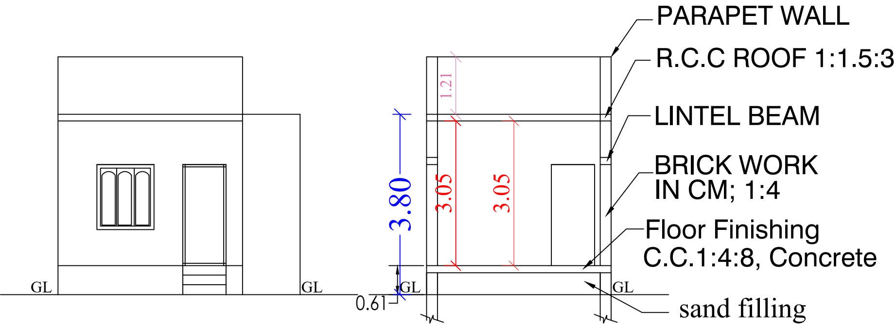
ELEVATION
