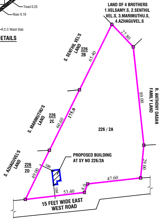
SITE PLAN (1:1000)
