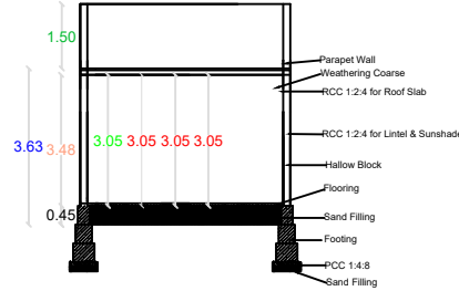
SECTION - AB
