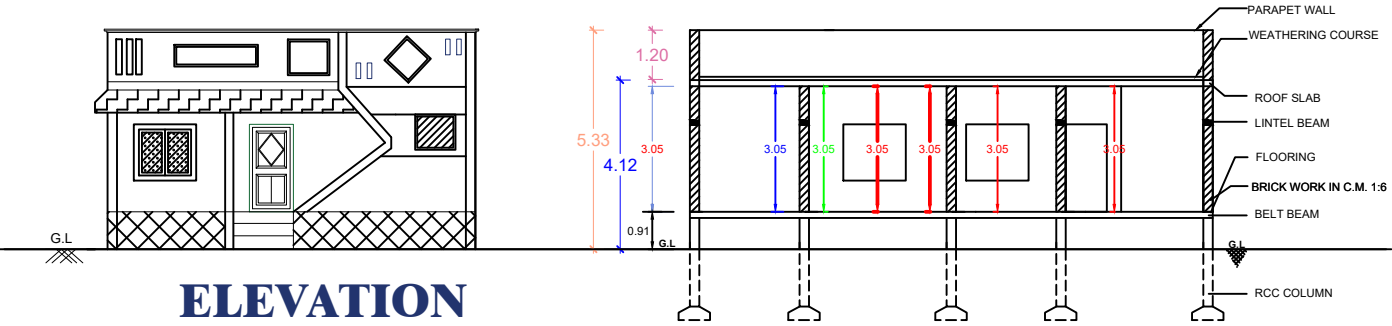
SECTION A-A
