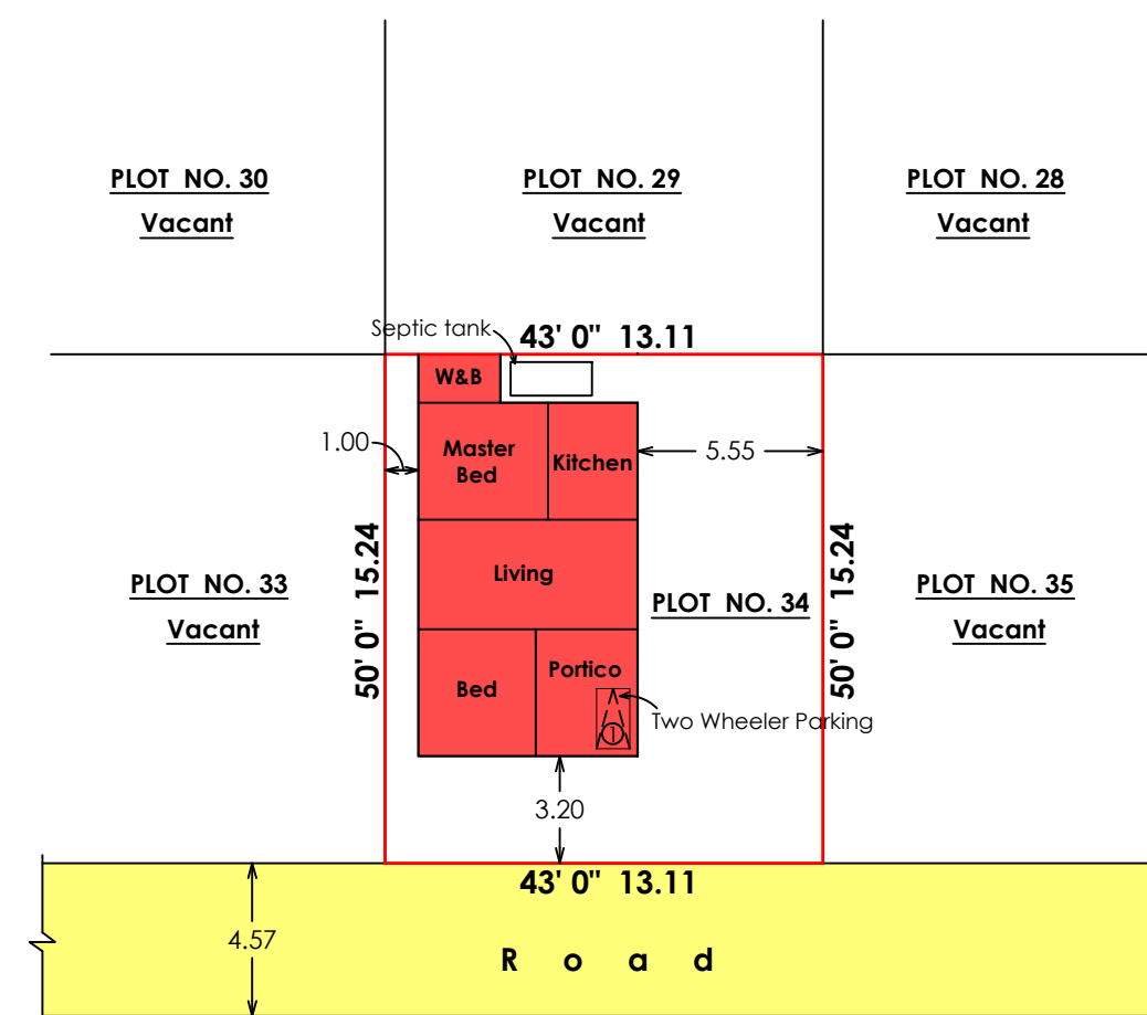
SITE PLAN SCALE - 1:250
