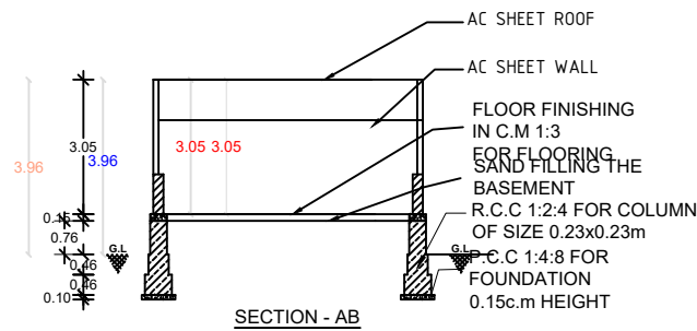
SECTION - AB
