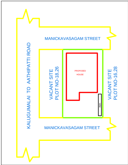
SITE PLAN (Scale 1:400)
