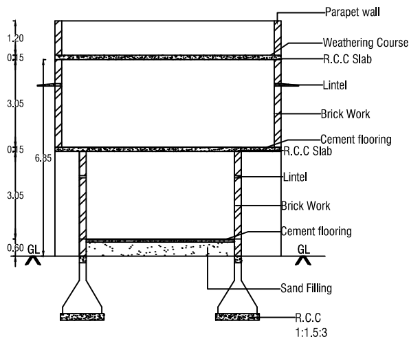
SECTION ON'AB'
