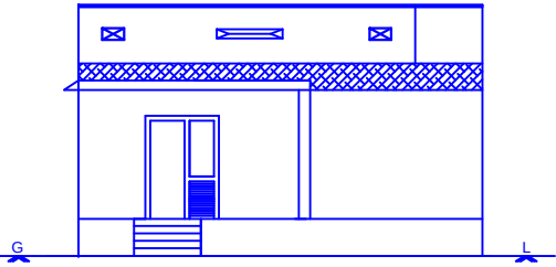
ELEVATION
