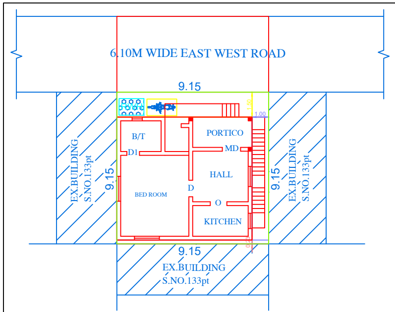
SITE PLAN(Scale 1 : 100)
