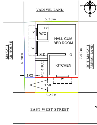
SITE PLAN ( SCALE : - 1:100 )
