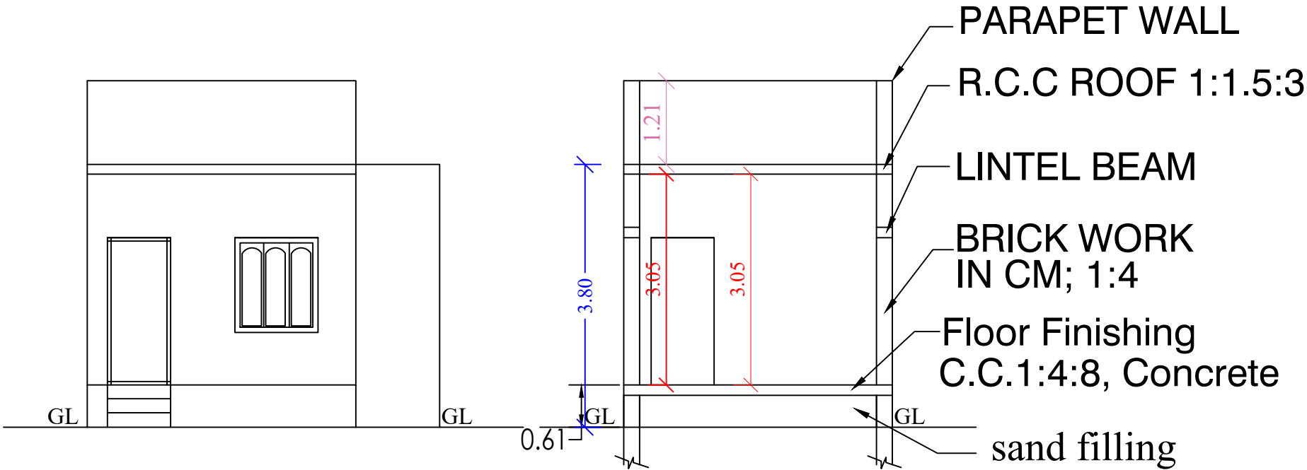
ELEVATION
