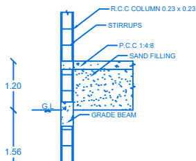
P.C.C 1:4:8
