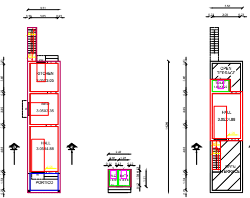
PRO. G.FLOOR PLAN
