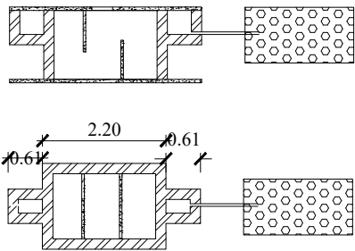
SEPTIC TANK & TRENCH - N.T.S
