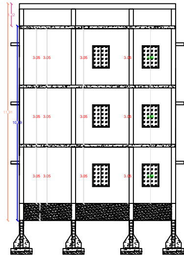
SECTION - AB
