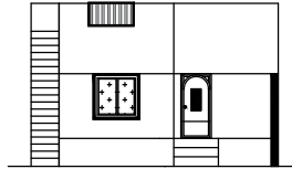
ELEVATION-A
