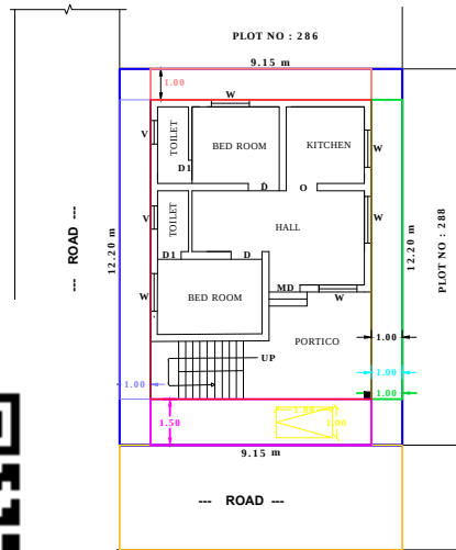
SITE PLAN ( 1:100 )
